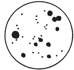
2. Pleiades
