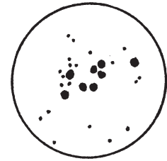
1. Pleiades
