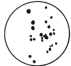
4. M7
