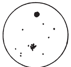
5. M13
