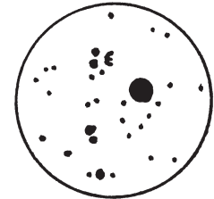
3. Coma Berenices
