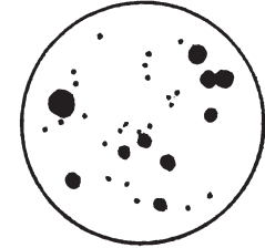
3. Pleiades
